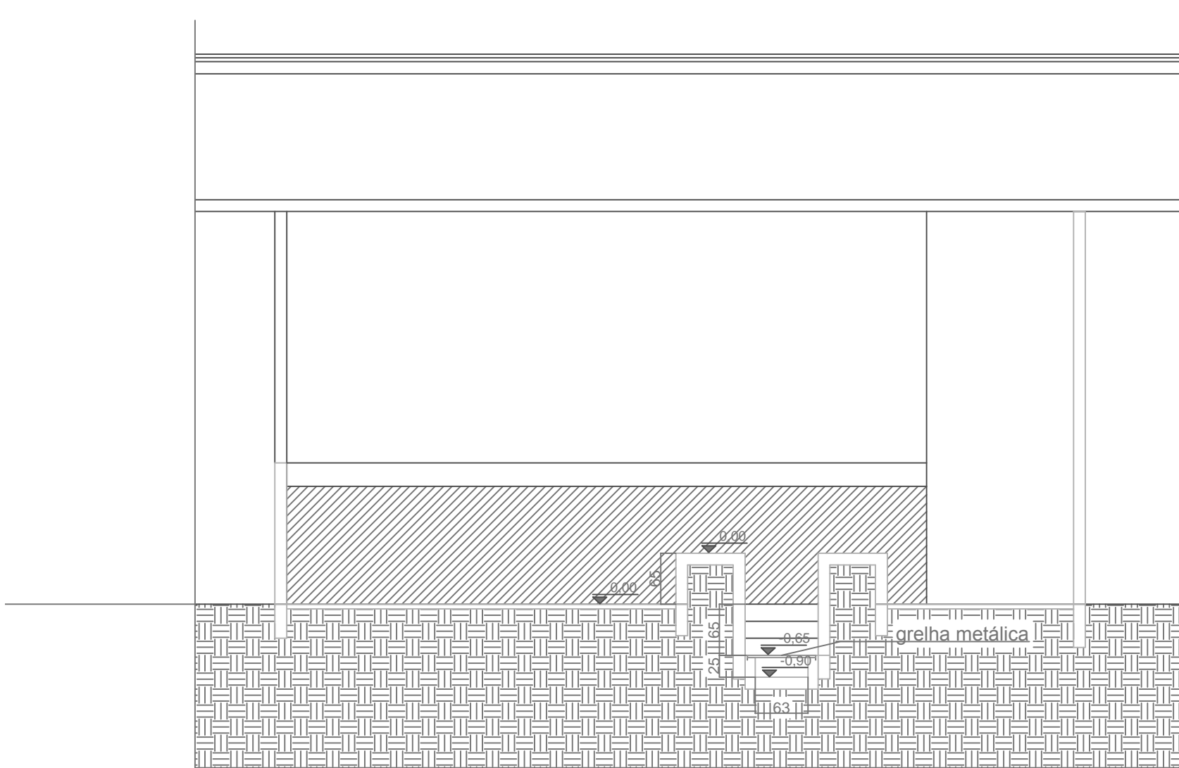
RAMPA DE LAVAGEM E TROCA DE ÓLEO CORTE C-C
