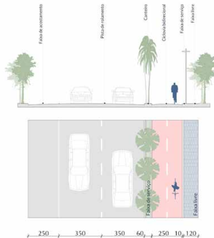
Perfil viário – Estrada principal com ciclovia
