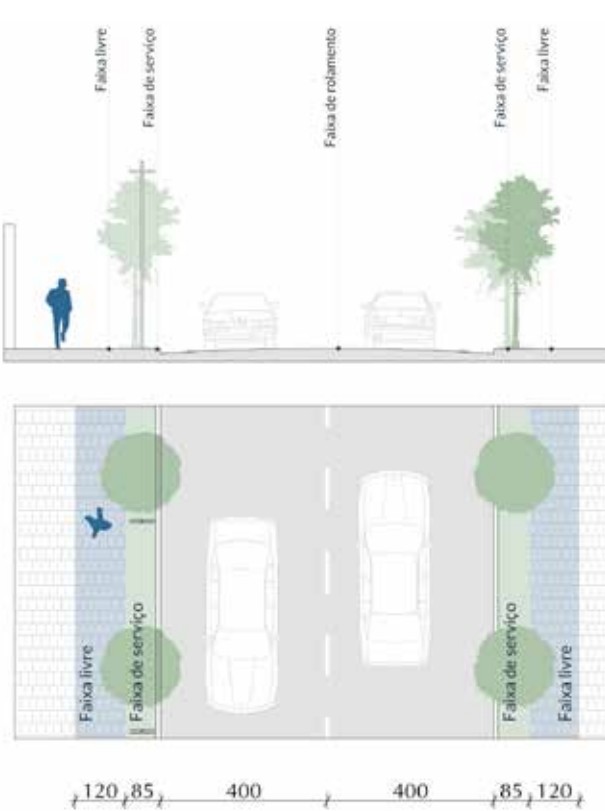
Perfil viário – Via estrutural sem ciclovia
