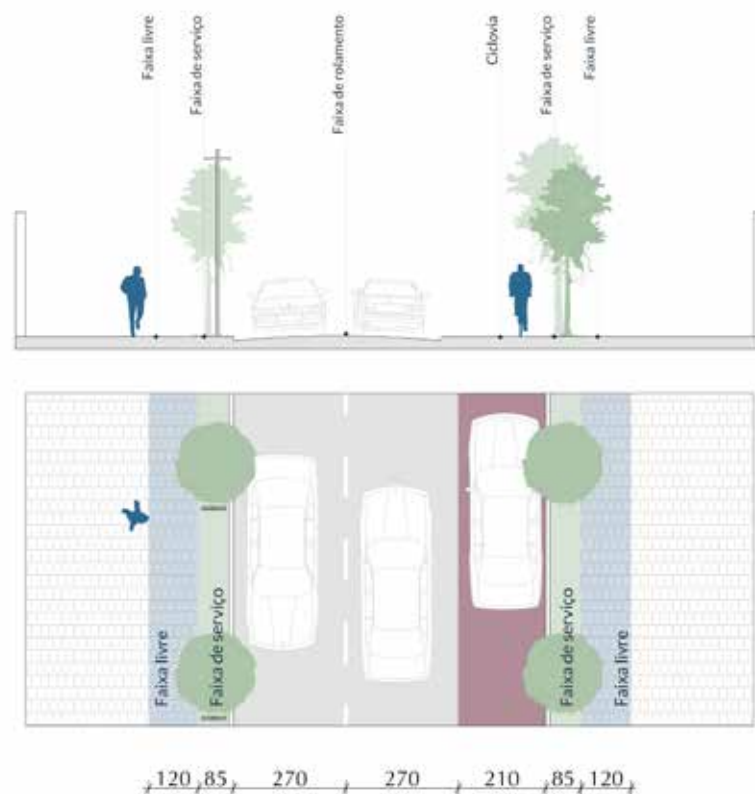
Perfil viário – Vias locais sem ciclovia
