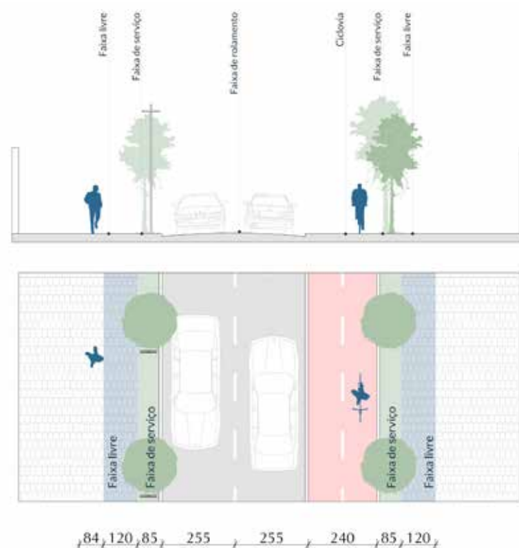
Perfil viário – Via local com ciclovia
