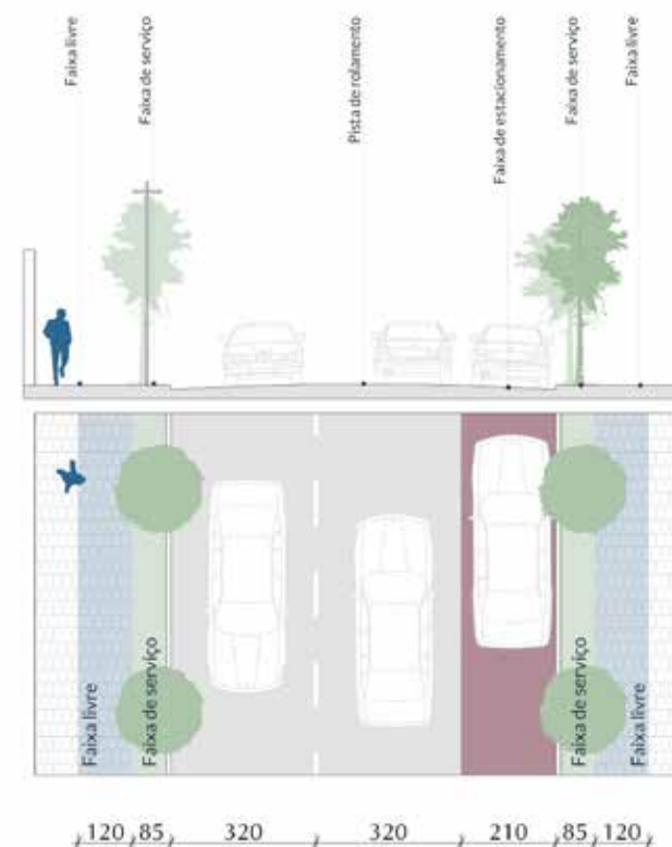
Perfil viário – Via conectora sem ciclovia
