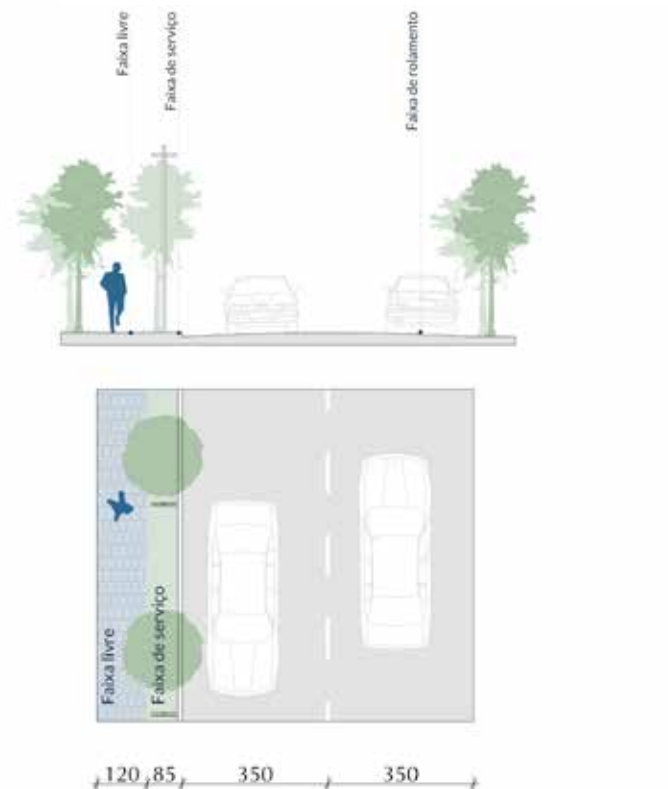
Perfil viário – Estrada vicinal sem ciclovia
