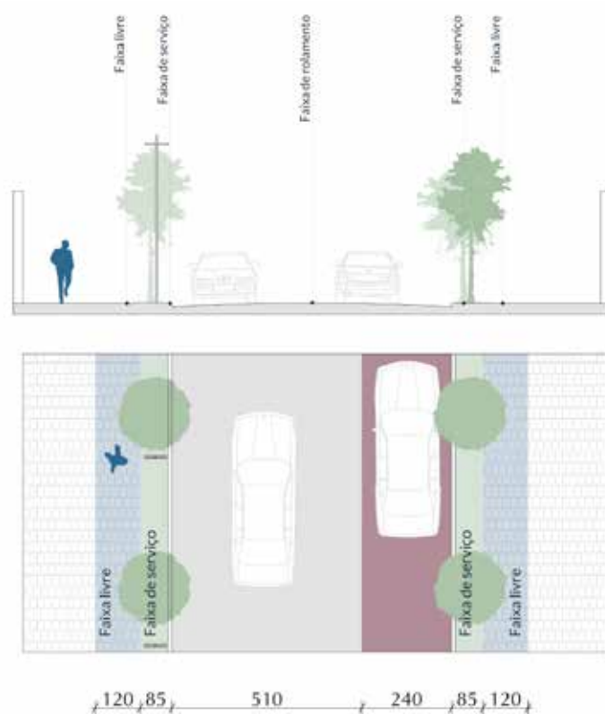
Perfil viário – Via especial unidirecional
