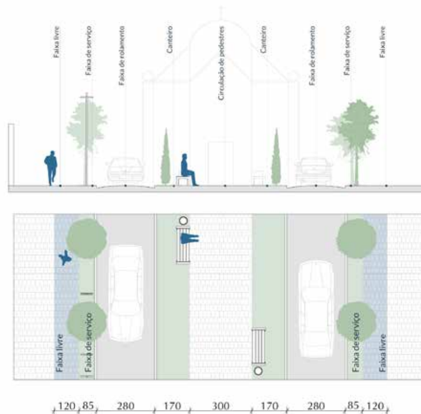
Perfil viário – Via especial com previsão de boulevard (Rua Conceição)
