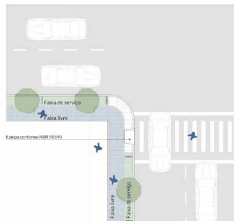
Esquinas – Via conectora sem ciclovia e via local sem ciclovia
