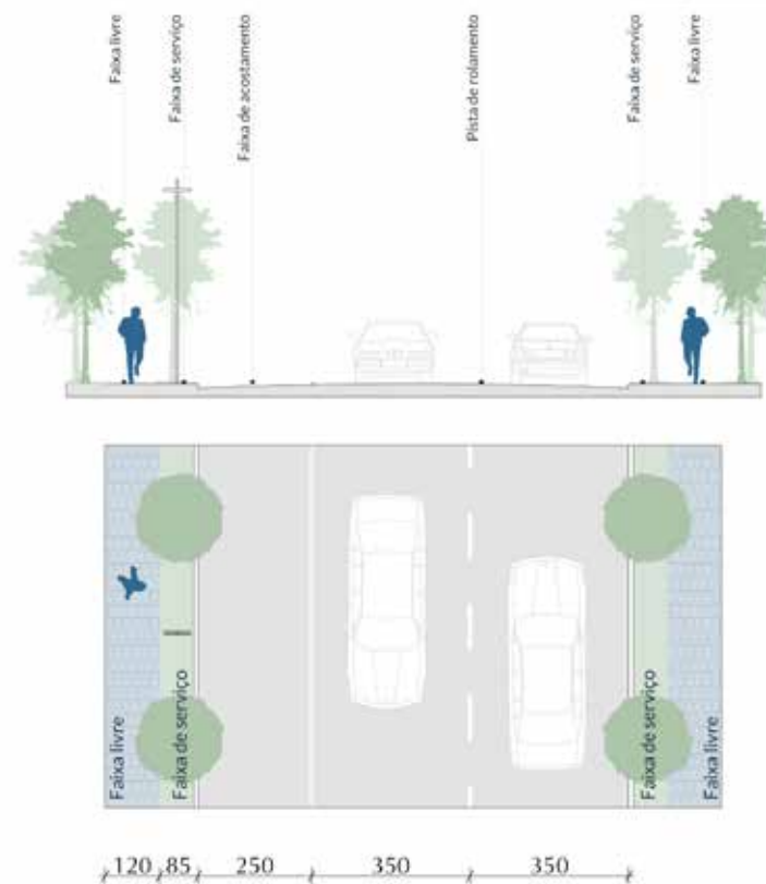
Perfil viário – Estrada principal sem ciclovia
