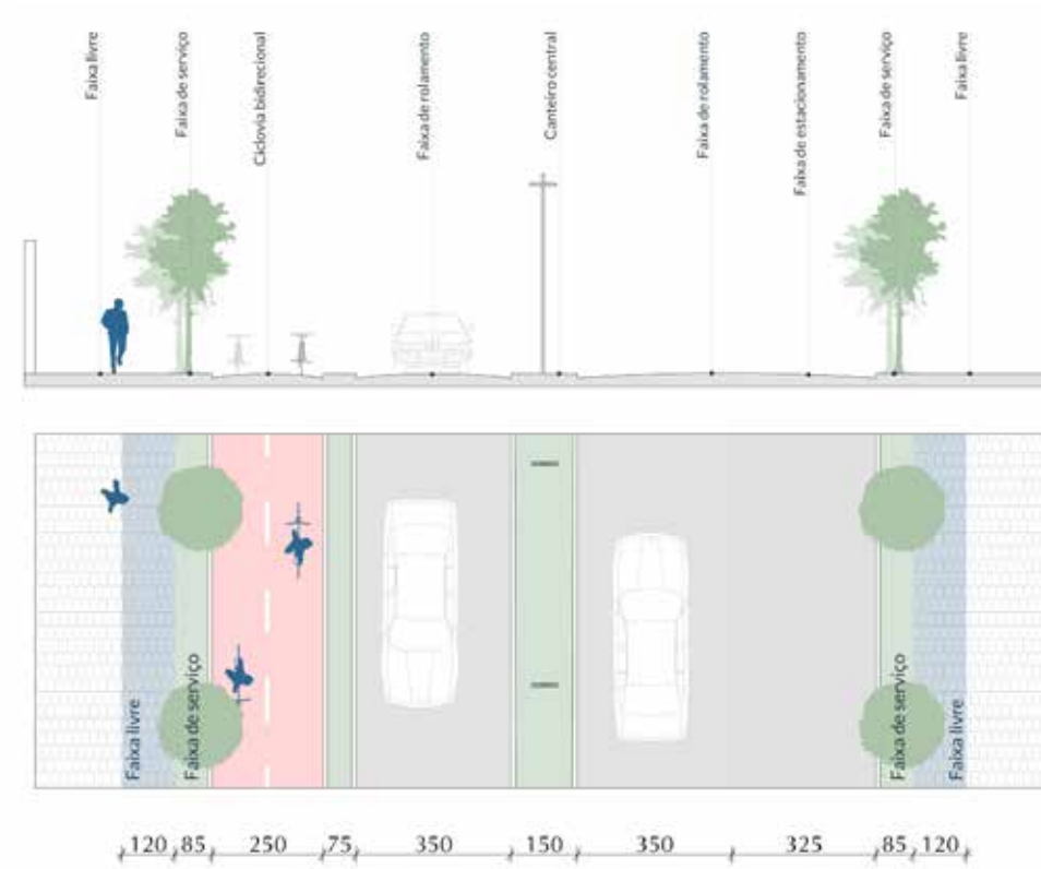
Perfil viário – Vias conectoras com ciclovia
